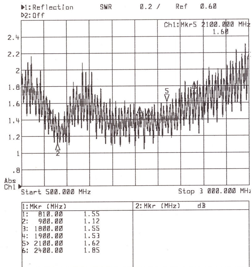
VSWR 500MHz – 3000MHz
