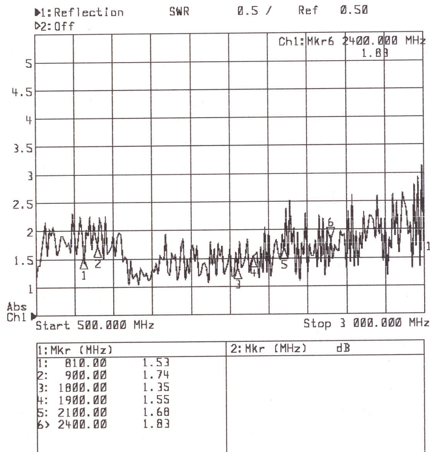
VSWR 500MHz – 3000MHz
