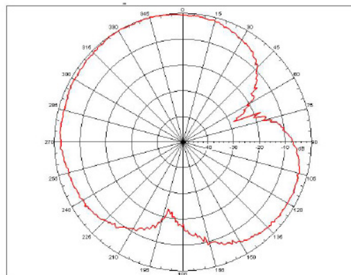
E-PLANE
