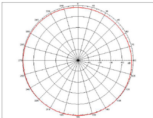
H-PLANE
